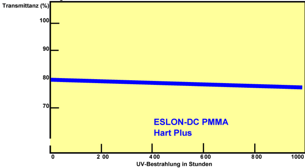
Lichtdurchlässigkeit
