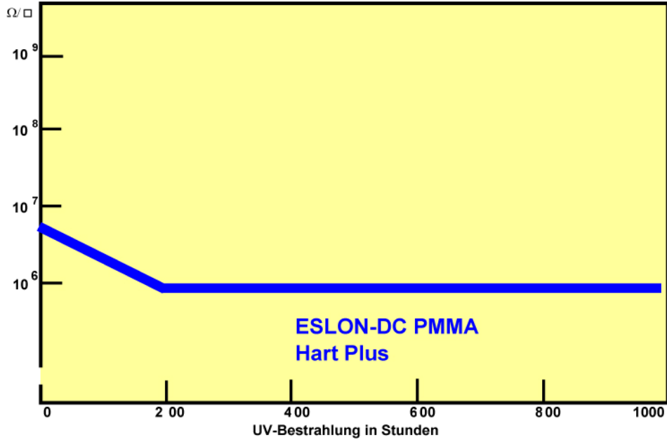
Oberflächenwiderstand
