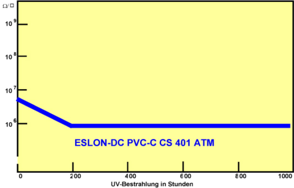
Oberflächenwiderstand
