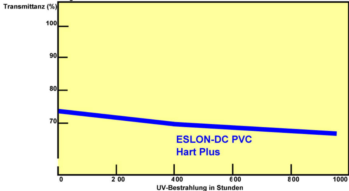
Lichtdurchlässigkeit
