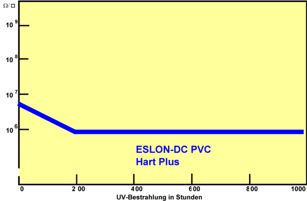
Oberflächenwiderstand
